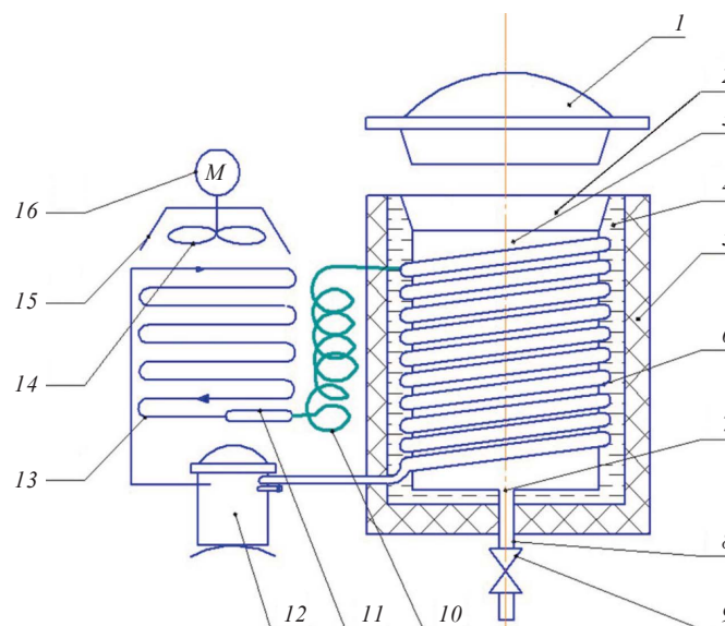
Рисунок 2. Схема криоконцентрактора емкостного типа (емкость 3,5 л). Криоконцентрактор состоит из теплоизолированной крышки – 1; заливной горловины – 2; цилиндрической емкости – 3, погруженной в хладоноситель – 4; теплоизоляции – 5; змеевика испарителя – 6; сливного отверстия – 7; трубопровода – 8; запорного вентиля – 9; капиллярной трубки – 10; фильтра осушителя – 11; компрессора – 12; воздушного конденсатора – 13; вентилятора – 14; кожуха – 15; электродвигателя вентилятора – 16
