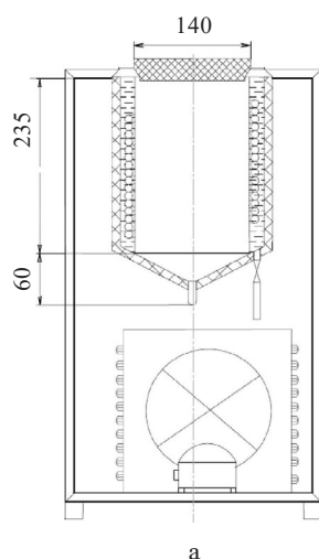
Рисунок 3. Конструкция криоконцентрактора: а – схема устройства; б – внешний вид
