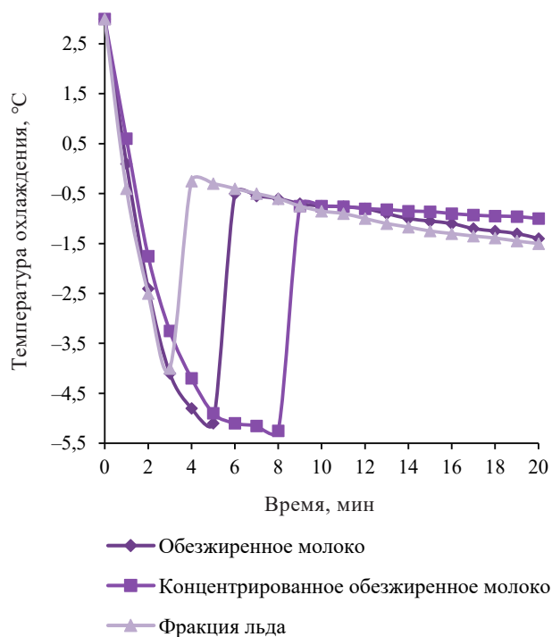
Рисунок 5. Кривые охлаждения
