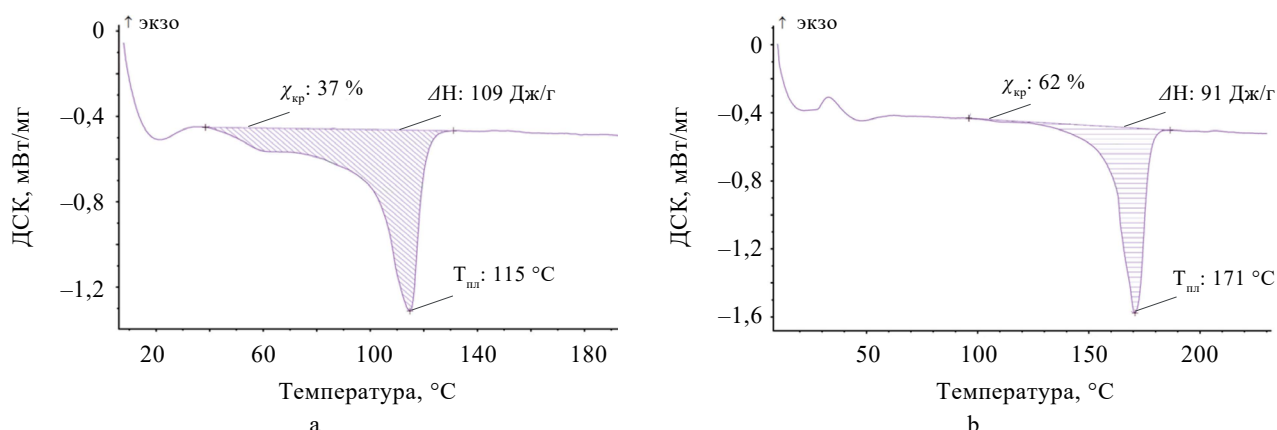
Рисунок 2. Теплофизические свойства полимерных композиций 90:10 мас. % при ультразвуковом воздействии: а – ПЭ:бетулин; б – ПП:бетулин
