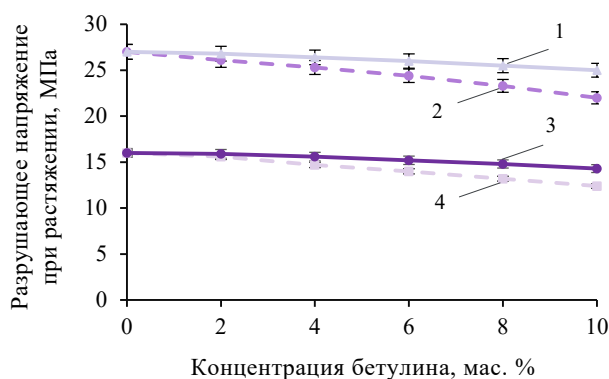
Рисунок 6. Влияние ультразвука на прочностные свойства полимерных композиций на основе полиолефинов, дисперсно-наполненных бетулином, при ультразвуковом воздействии (1 – ПП, 3 – ПЭ); без ультразвукового воздействия (2 – ПП, 4 – ПЭ)
